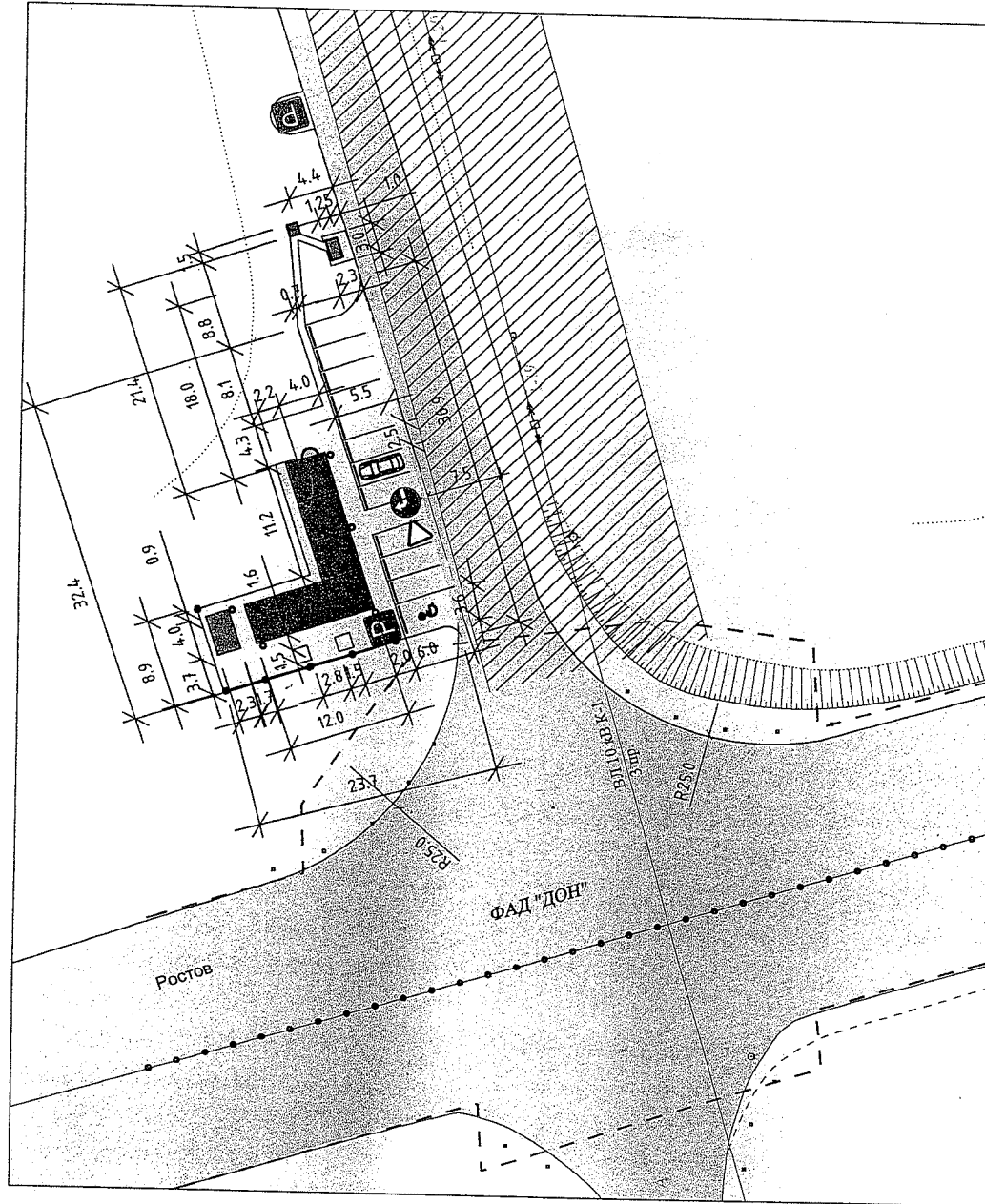
Ситуационный план
