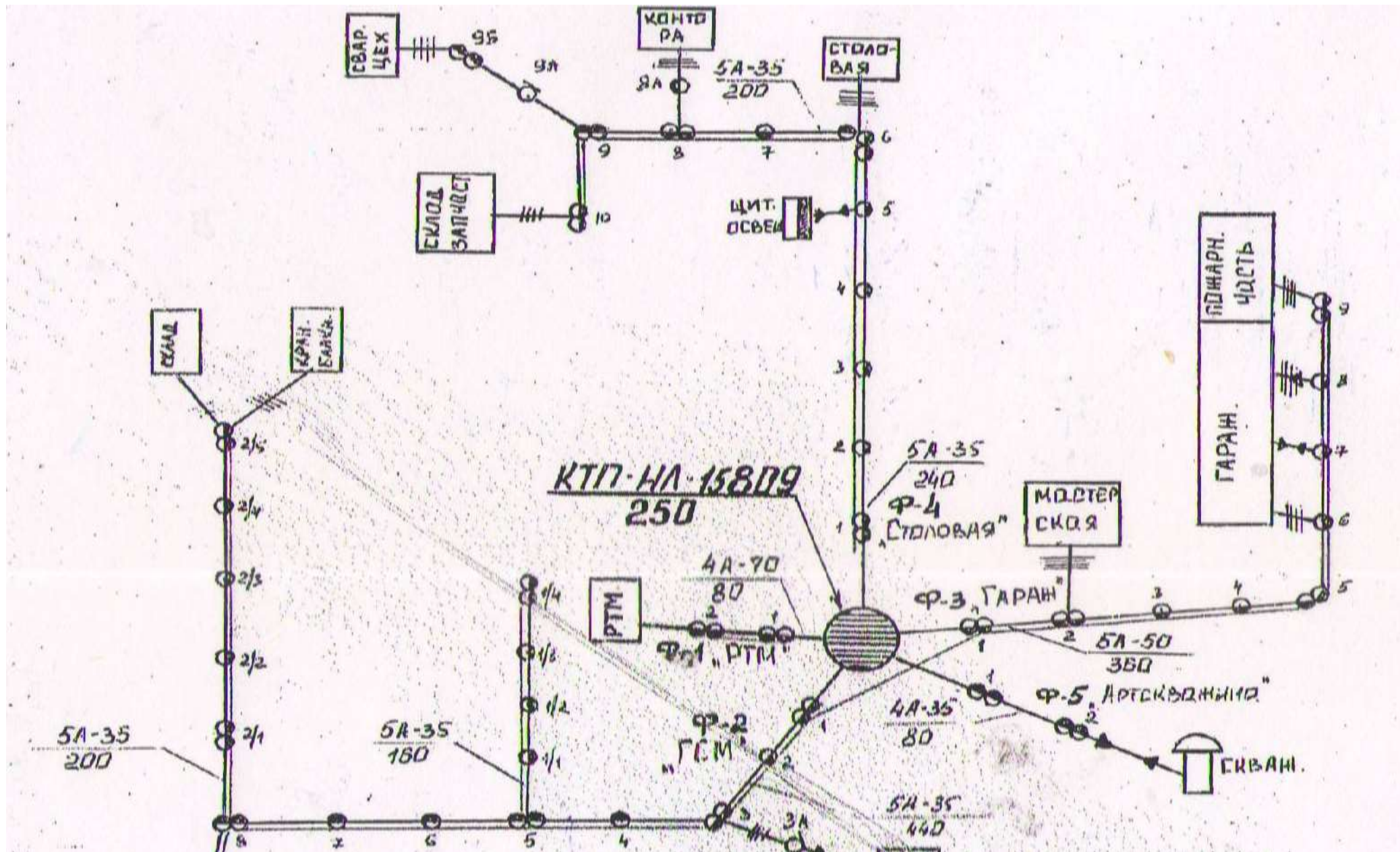
Обосновывающие материалы. Схема электроснабжения (лист № 9) ст. Новолешковская. Масштаб 1:5000
