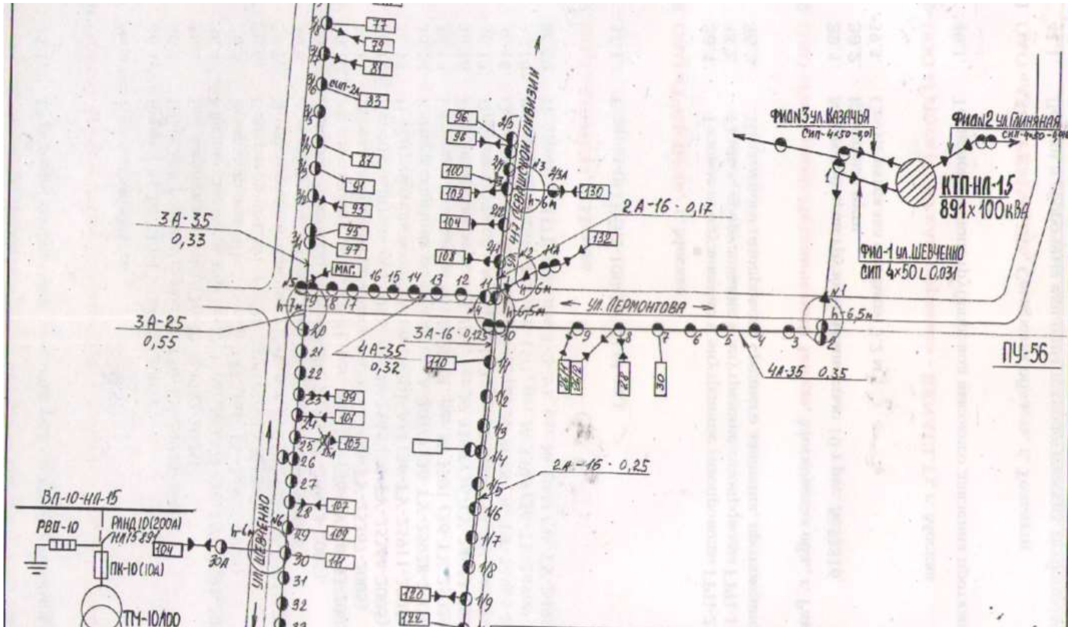
Обосновывающие материалы. Схема электроснабжения (лист № 54) ст. Новолешковская. Масштаб 1:5000
