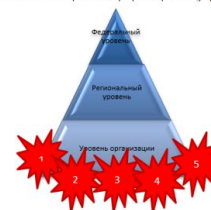
Рисунок 3. Пирамида проблем
