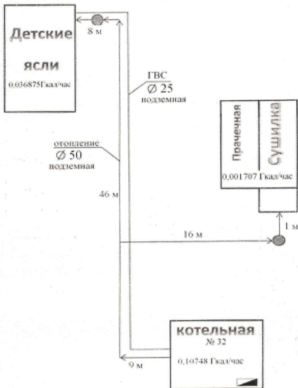
Рисунок 25 Карта (схема) тепловых сетей в зоне действия котельной № 32
