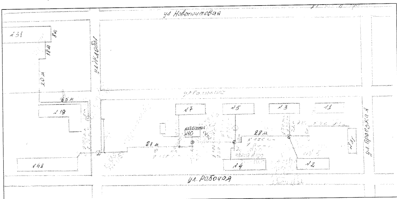
Рисунок 13 Схема теплотрассы от котельной № 10 ст. Павловская
