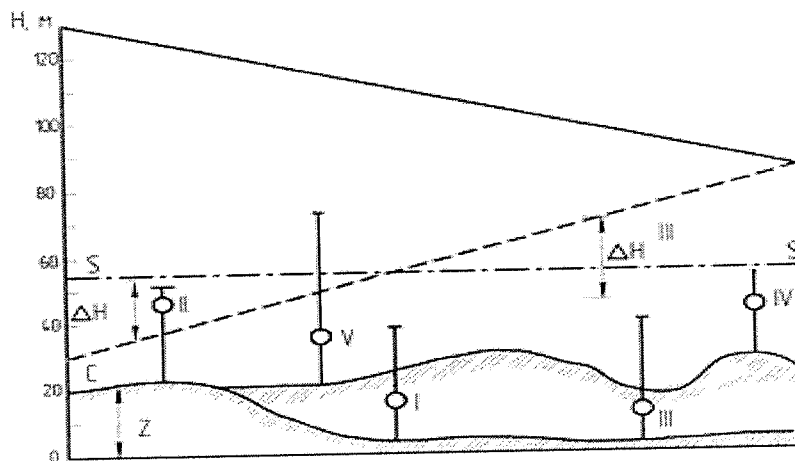
Рисунок 27 Пьезометрический график тепловых сетей
