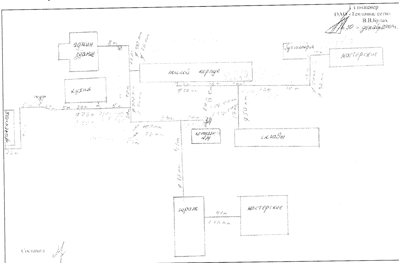
Рисунок 17 Схема теплотрассы от котельной № 14 ст. Павловская
