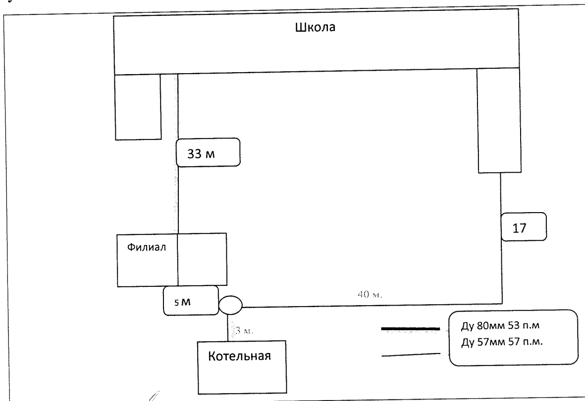
Рисунок 19 Схема теплотрассы от котельной № 25 ст. Павловская
