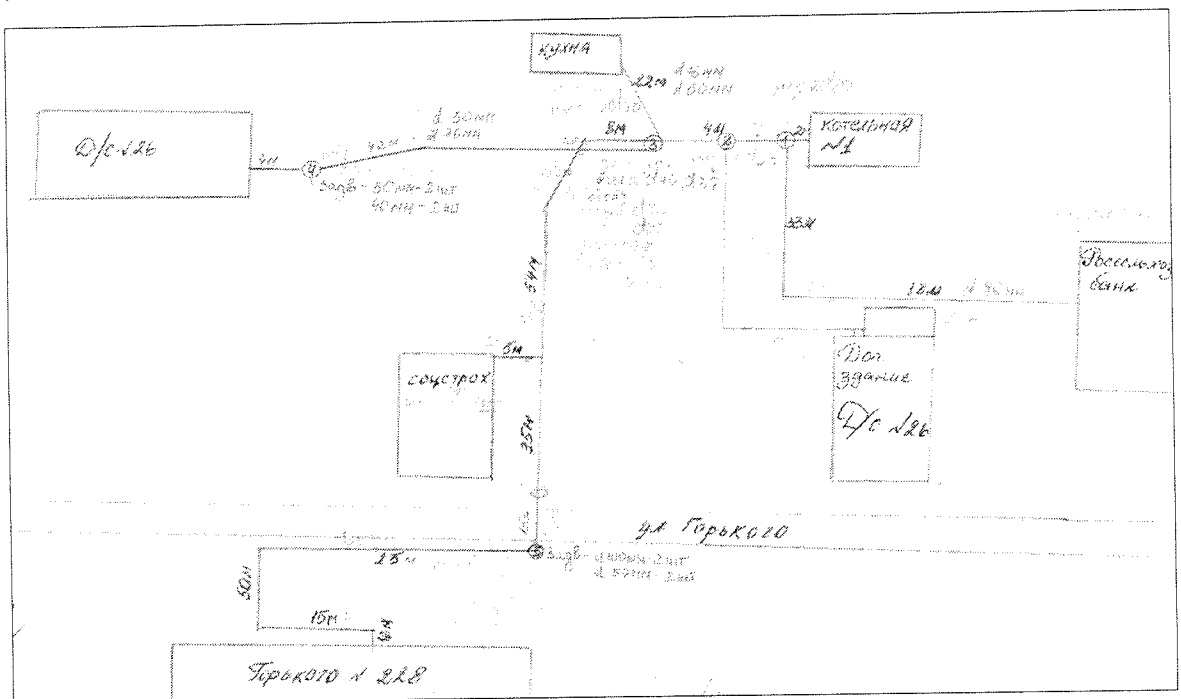
Рисунок 5 Схема теплотрассы от котельной № 1 ст. Павловская
