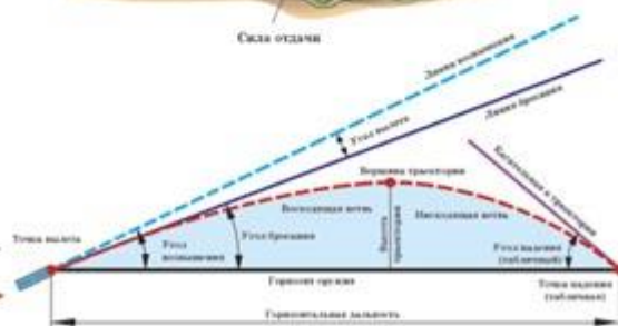
Элементы траектории полёта пули
