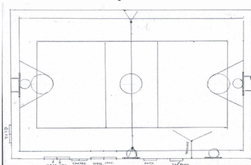
Схема спортивного зала
