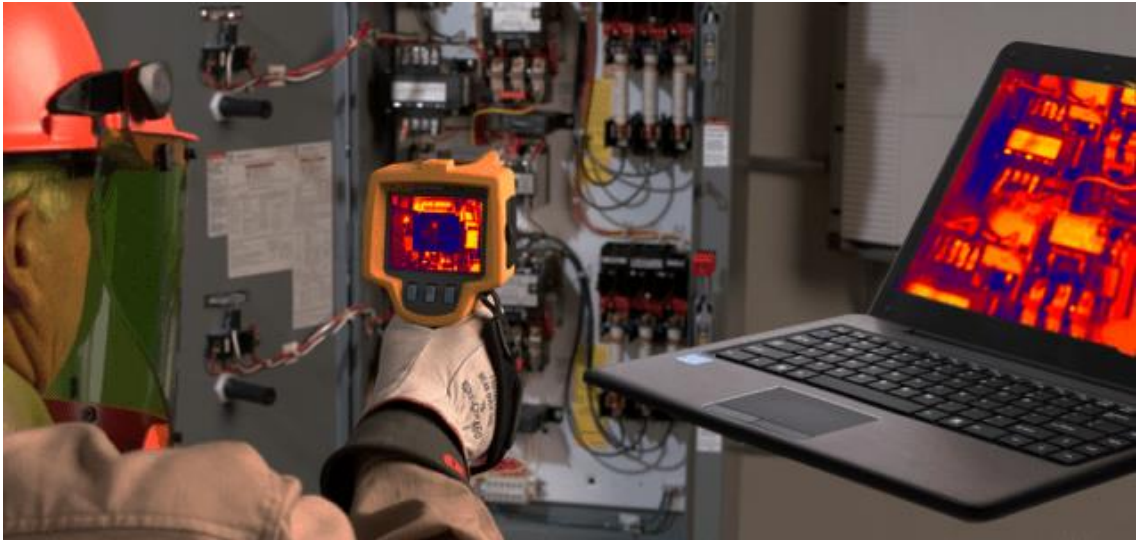
Рисунок 20. Пример проведения тепловизионного контроля электрошкафа
