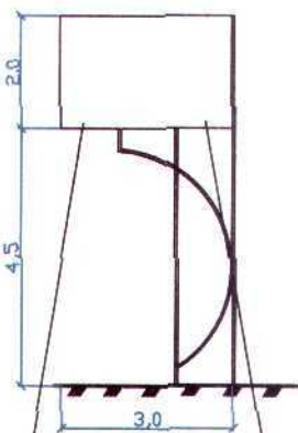
Эскиз рекламной конструкции
