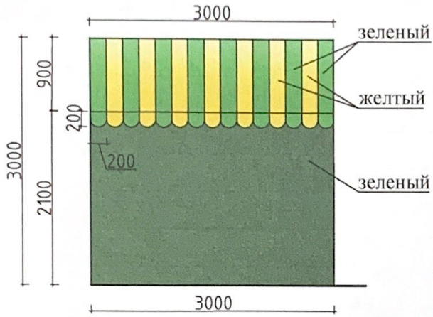
Вид спереди
