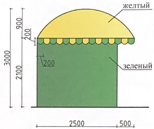
Вид сбоку
