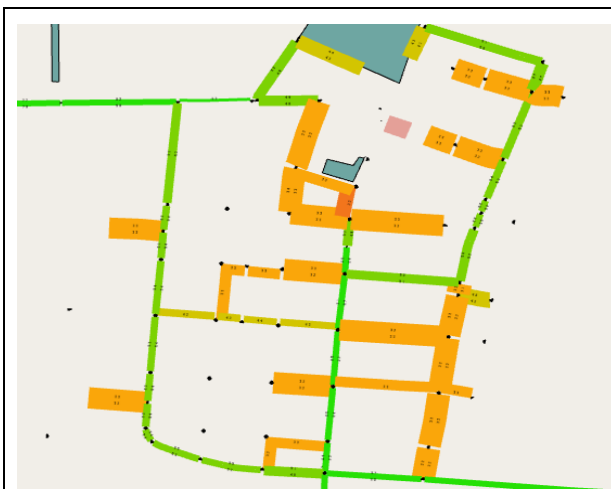
Рисунок 19 Картограмма уровней скоростного обслуживания ст.Новосергиевская
