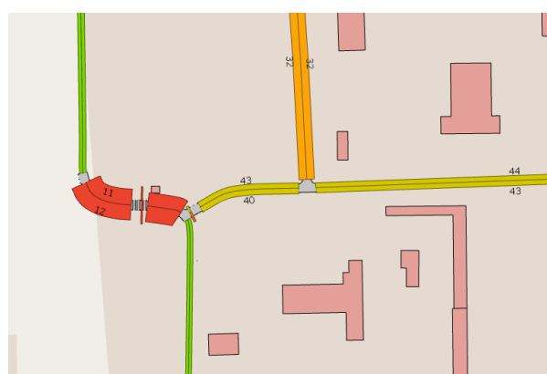
Рисунок 18 Картограмма уровней скоростного обслуживания на железнодорожном переезде по ул.Красногвардейская в ст-це Октябрьская
