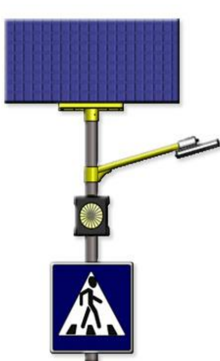
Рисунок 58 Комплект освещения пешеходного перехода на солнечных электростанциях
