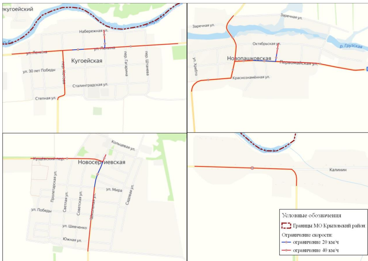
Рисунок 50 Расположение планируемых зон успокоенного движения (3)
