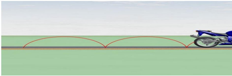
Рис. 2 – Циклоида как траектория движения точки катящегося колеса
