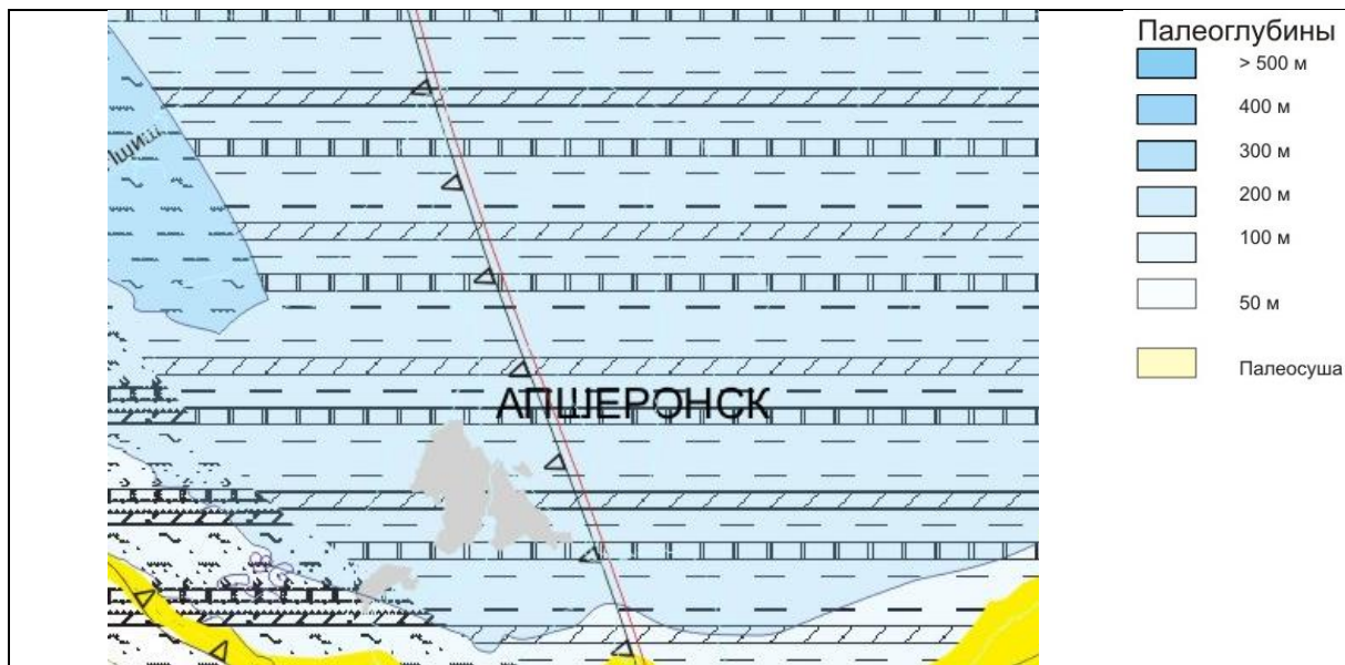
Рис. 1 - Палеогеографическая схема раннесарматского бассейна у г. Апшеронск
