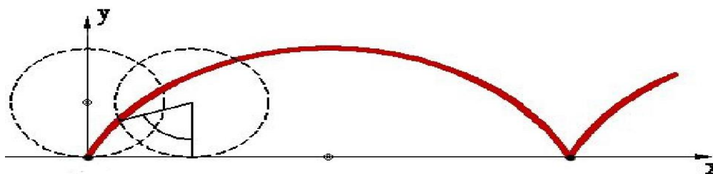
Рис. 1 – Так выглядит циклоида на графике
