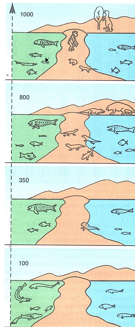
Рис. 63. Компьютерное моделирование эволюционного процесса
