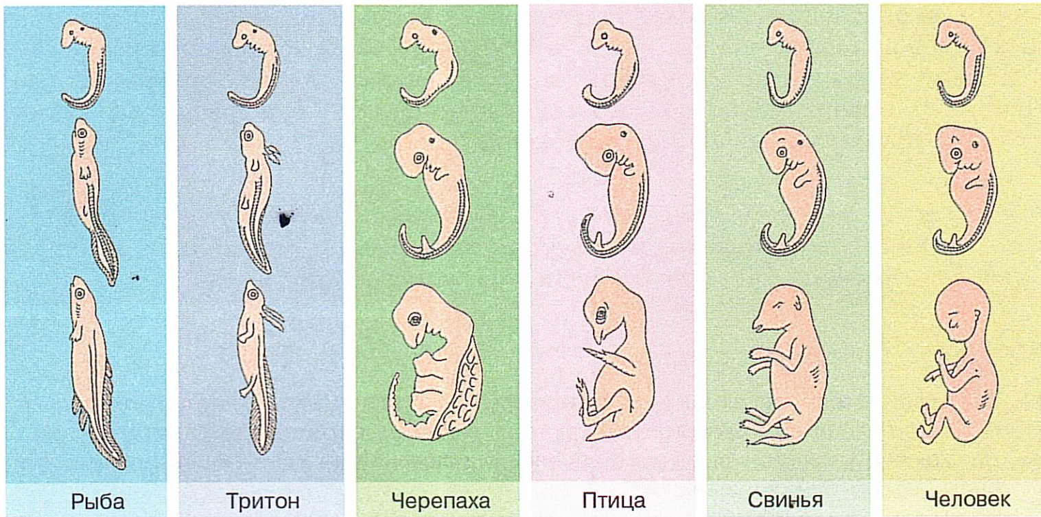
Рис. 50. Зародыши различных классов позвоночных животных
