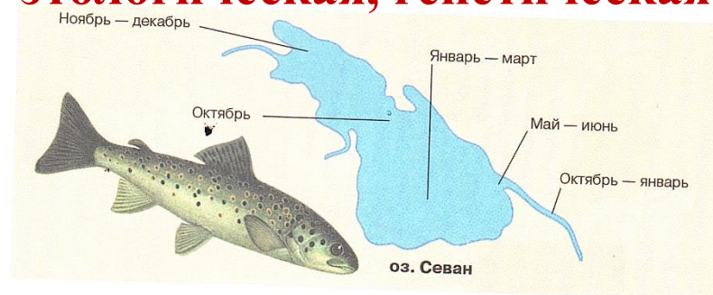
Рис. 24. Экологическая изоляция пяти популяций севанской форели (показаны места обитания популяций в озере, различающихся сроками нереста)
