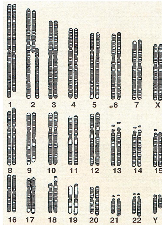
Рис. 62. Схематические карты дифференциально окрашенных хромосом человека и шимпанзе (первые хромосомы в парах — человека, вторые — гомологичные им — шимпанзе; во 2-й паре две хромосомы у шимпанзе идентичны одной хромосоме человека, которая является результатом их слияния)
