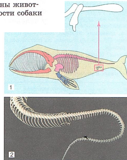
Рис. 58. Рудименты: 1 — тазового пояса кита; 2 — конечностей питона
