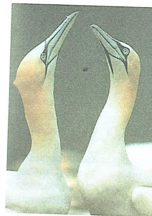
Рис. 25. Оpozнание партнёра во время брачного ритуала у олушей
