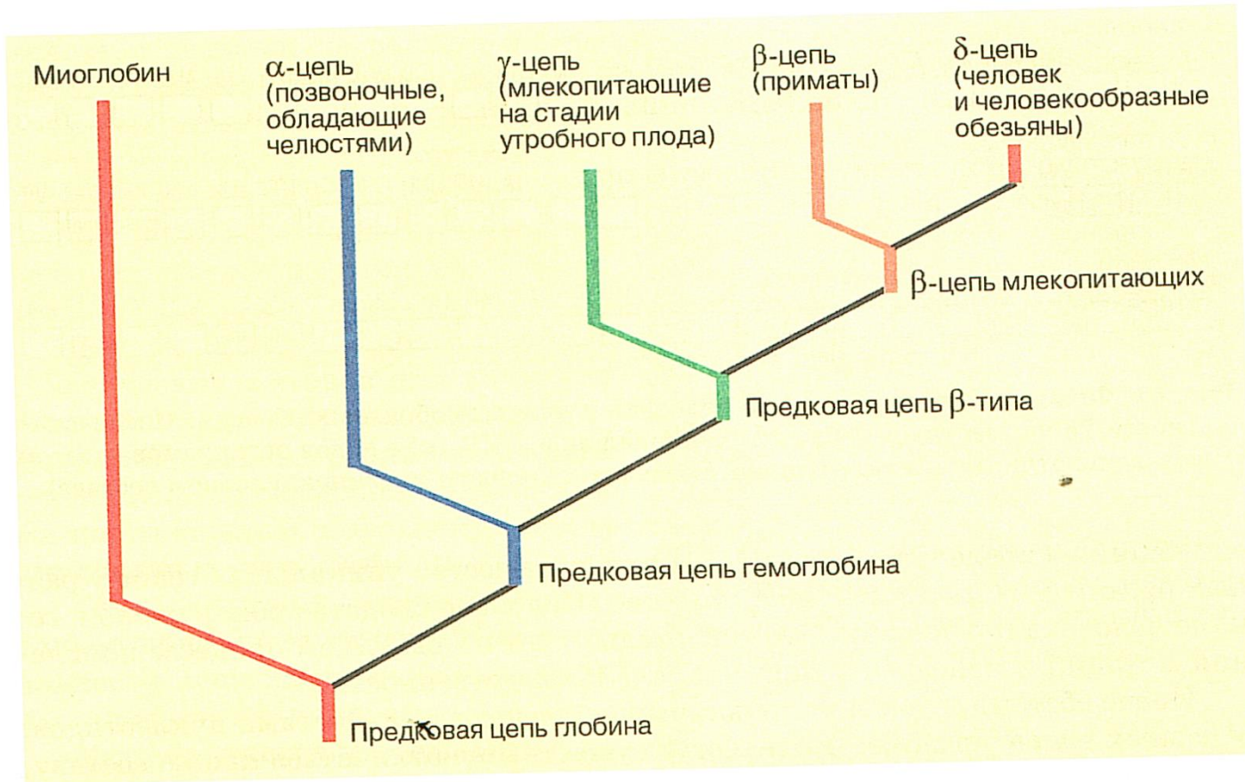
Рис. 60. Схема происхождения миоглобина и гемоглобина у позвоночных животных
