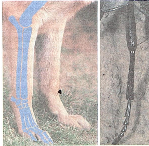
Рис. 55. Аналогичные органы животных — бегательные конечности собаки и жука
