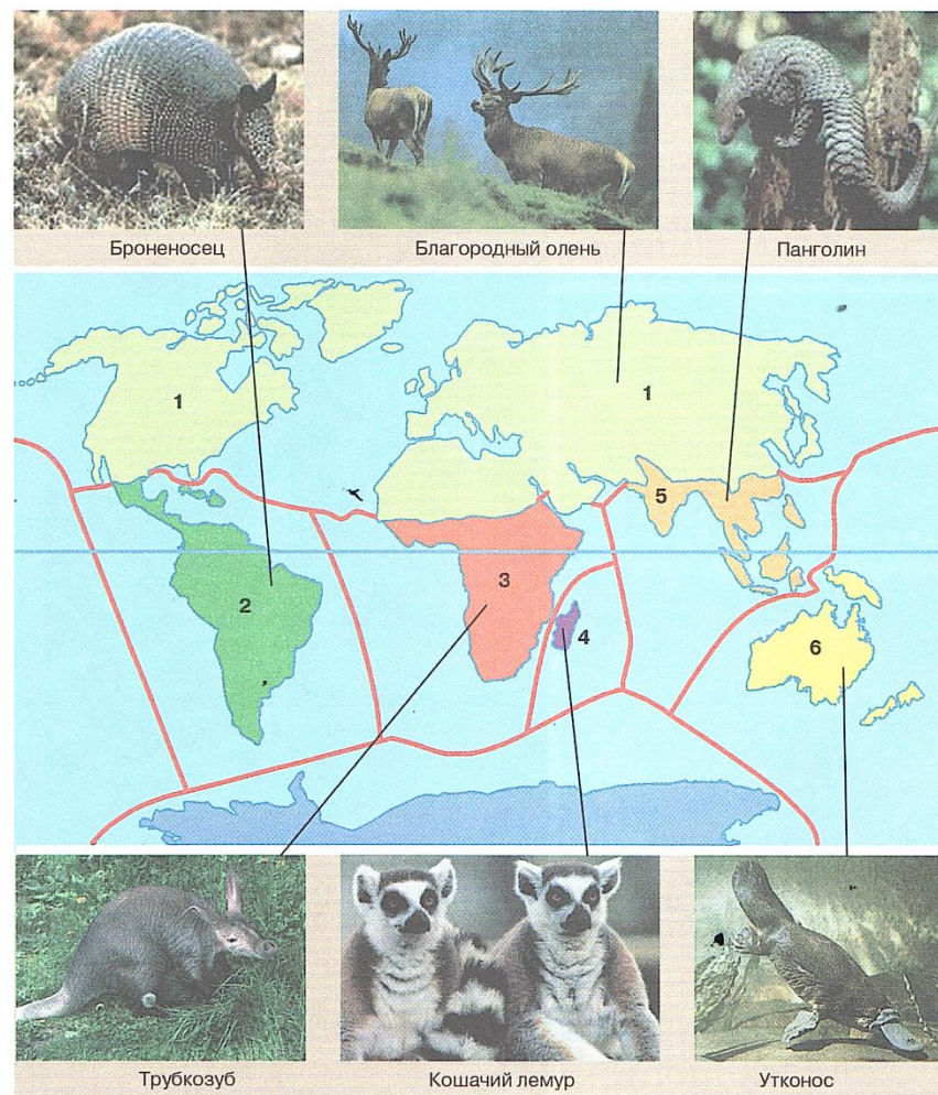
Рис. 48. Биogeографические области Земли и их млекопитающие — эндемики: 1 — Голарктическая; 2 — Неотропическая; 3 — Эфиопская; 4 — Мадагаскарская; 5 — Индо-Малайская; 6 — Австралийская
