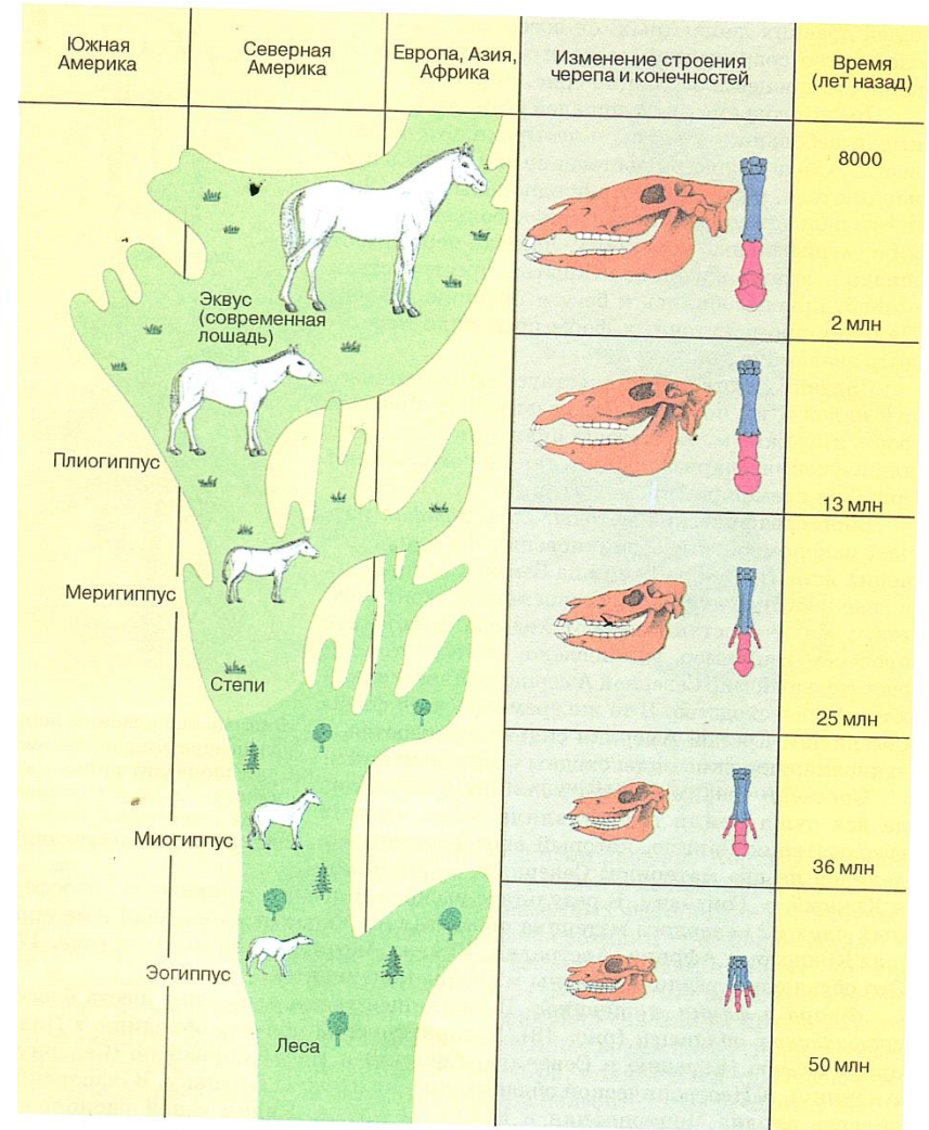
Рис. 46. Эволюционное древо семейства Лошадиные
