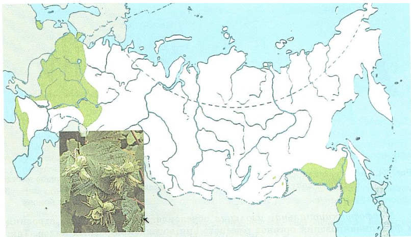
Рис. 23. Географическая изоляция популяций внутри ареала лещины обыкновенной
