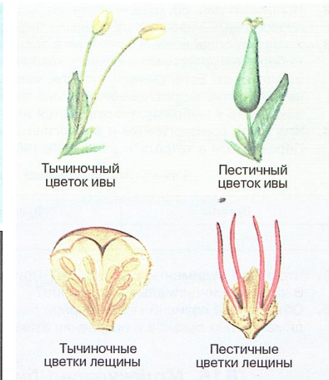
Рис. 59. Рудименты у растений — редуцированные околоцветники
