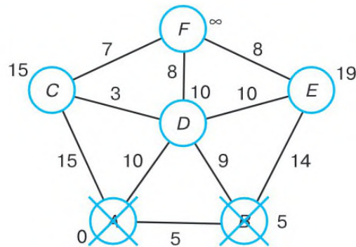
Рис. 3.14. Алгоритм Дейкстры. Шаг 2
