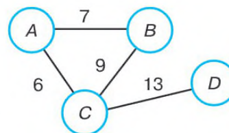
Рис. 3.5. Граф схемы дорог
