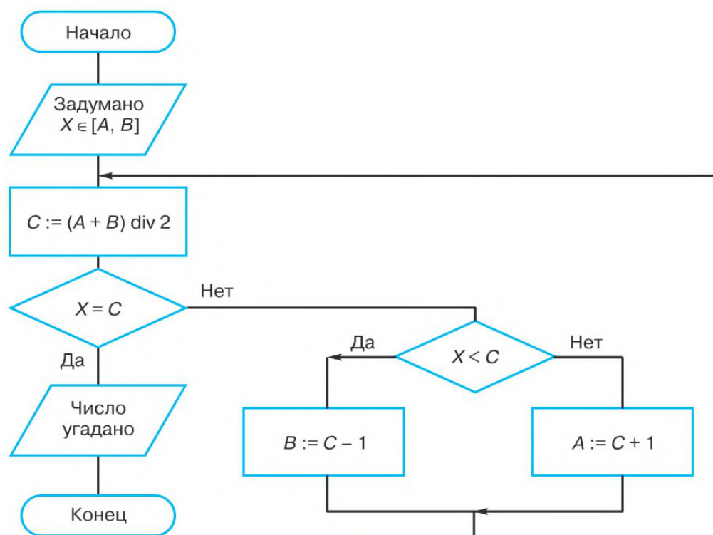
Рис. 2.3. Метод половинного деления
