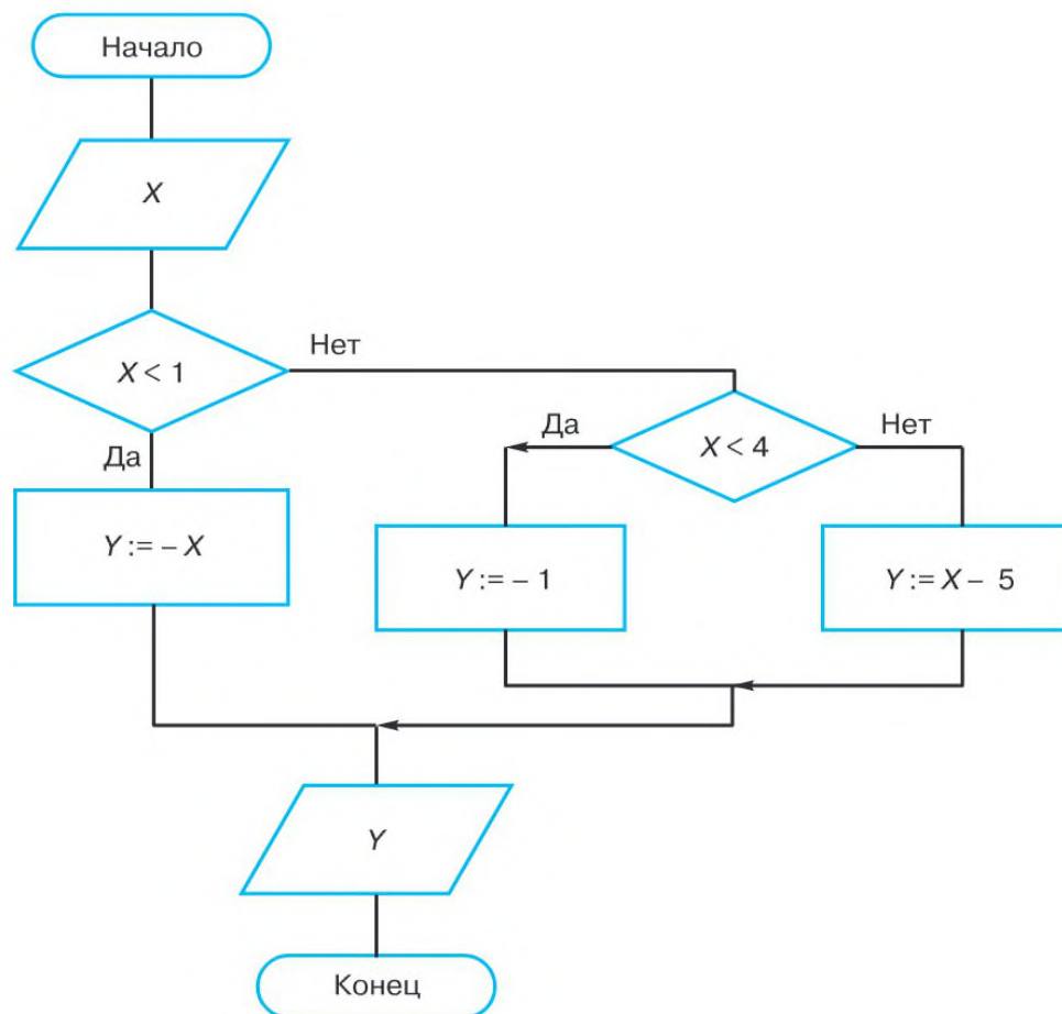
Рис. 2.7. Алгоритмическая конструкция «ветвление»
