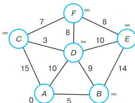
Рис. 3.12. Алгоритм Дейкстры. Начальное состояние
