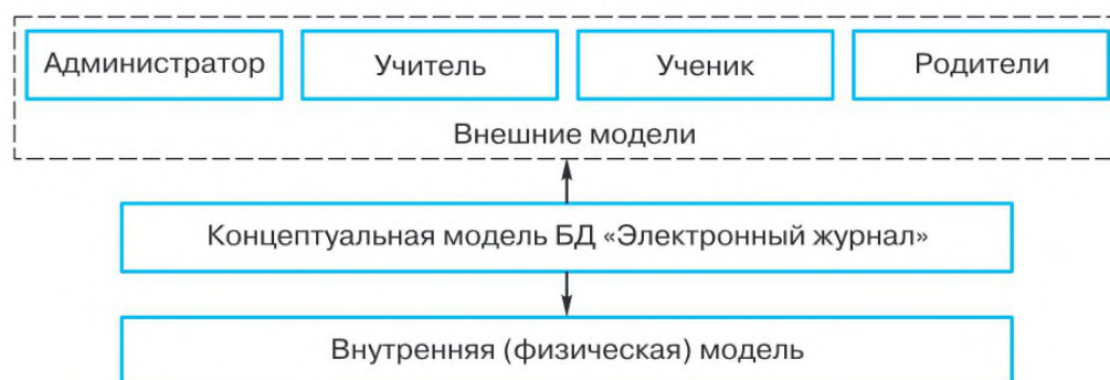
Рис. 3.30. Уровни представления данных БД «Электронный журнал»
