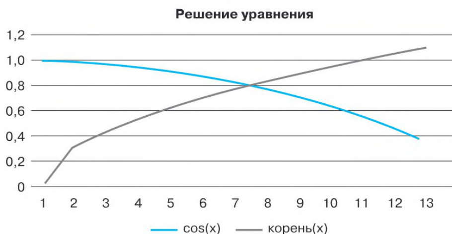
Рис. 1.13. Графики функций
