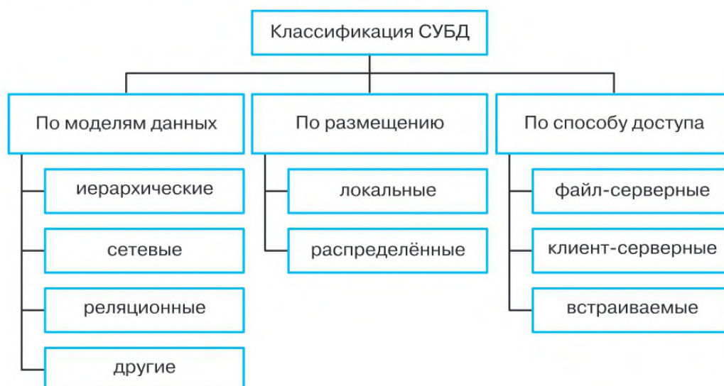
Рис. 3.31. Классификация СУБД
