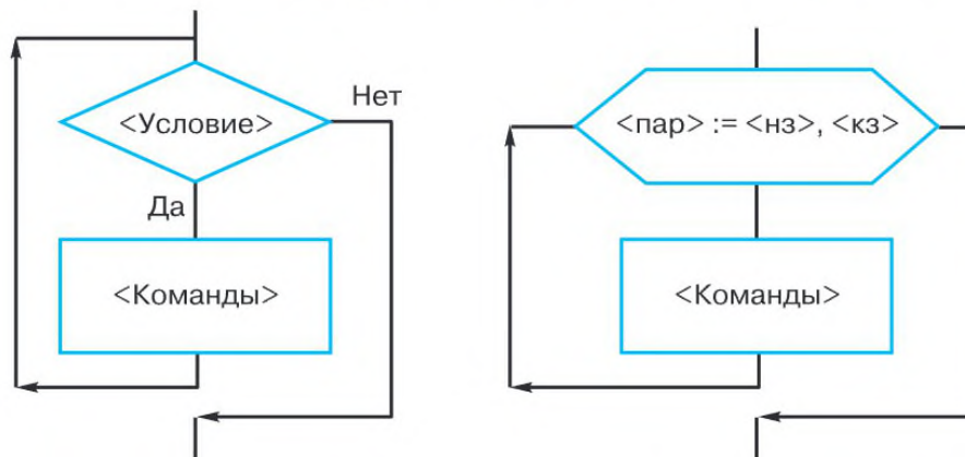
Рис. 2.8. Блок-схемы циклов
