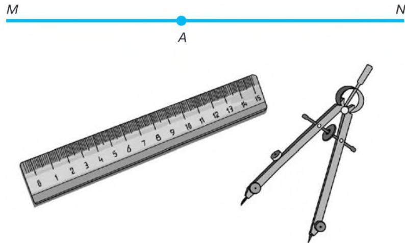
Рис. 2.2. Построение перпендикуляра к прямой
