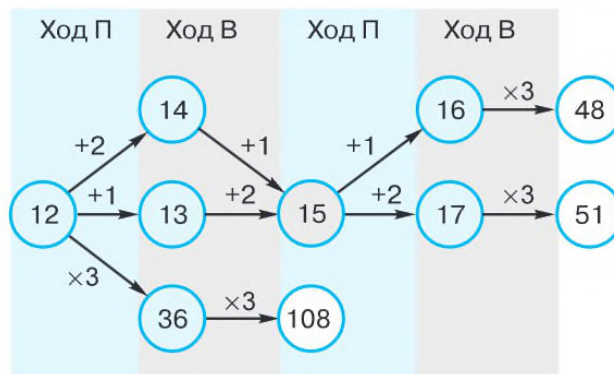
Рис. 3.21. Позиция 12 — проигрышная для Пети
