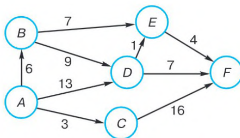
Рис. 3.7. Ориентированный граф
