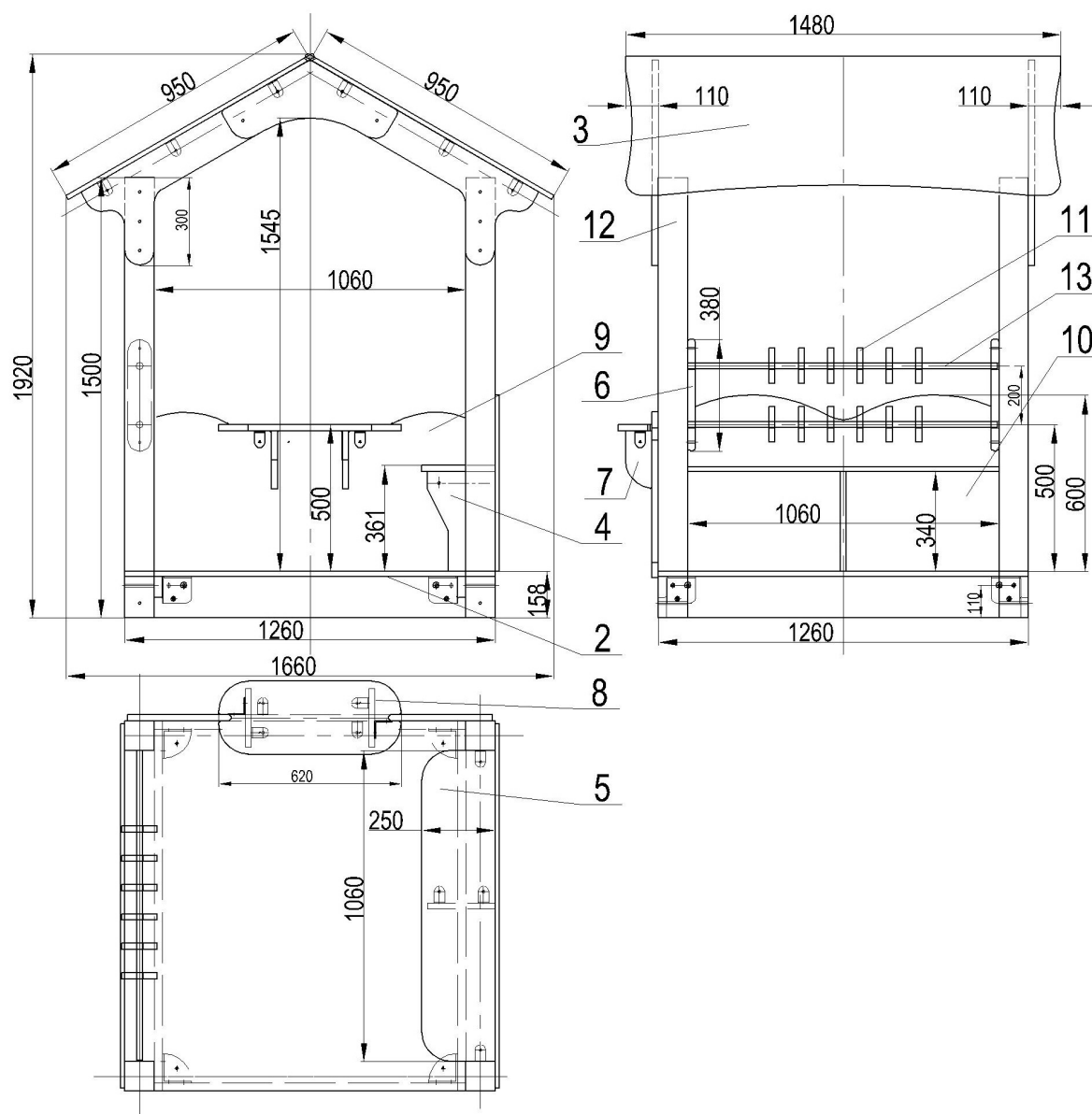
Общий вид детского игрового оборудования.
