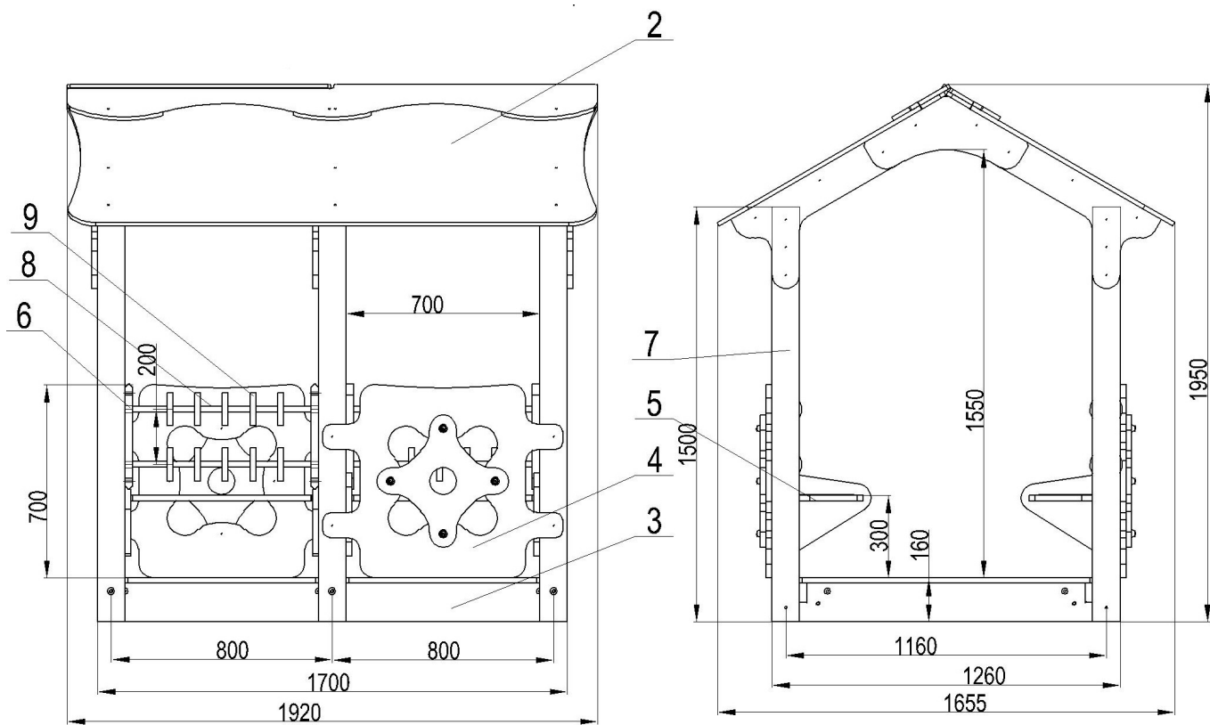
Общий вид детского игрового оборудования.
