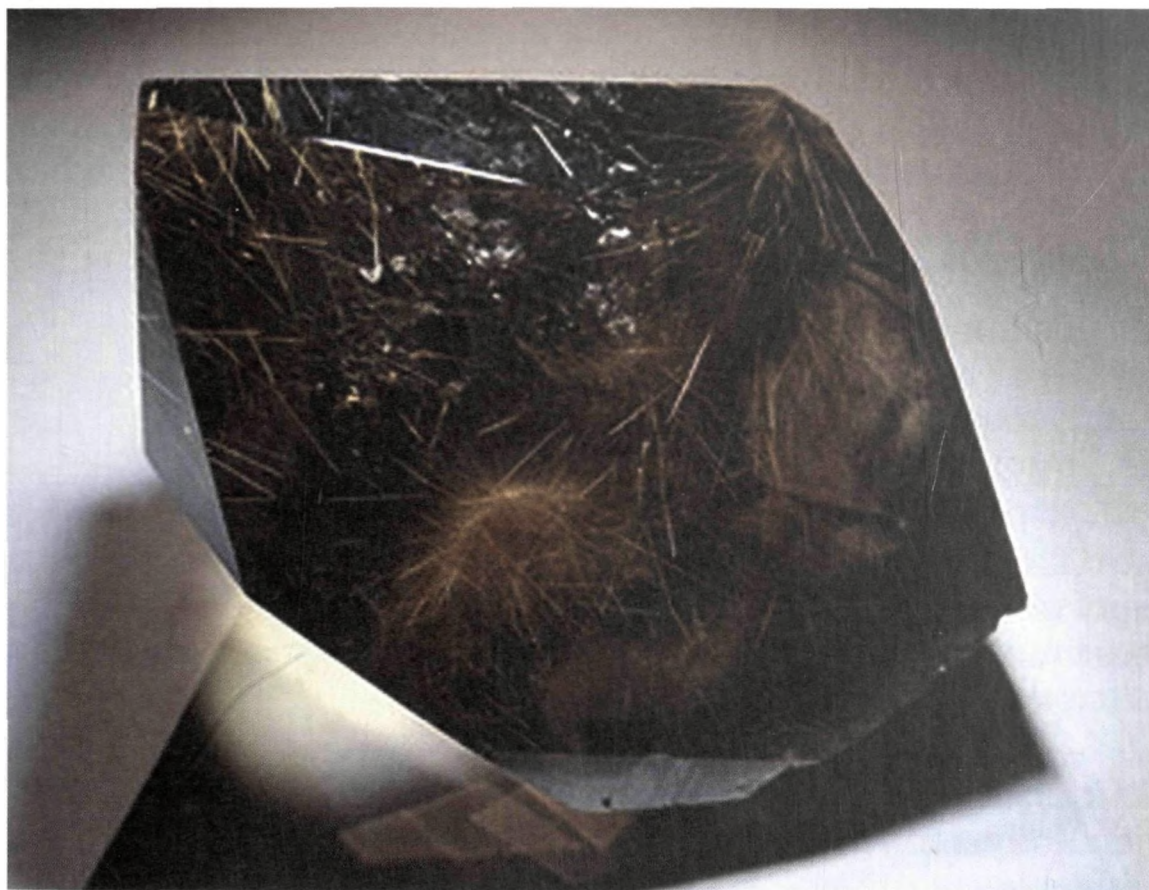
Кварц-волосатик
