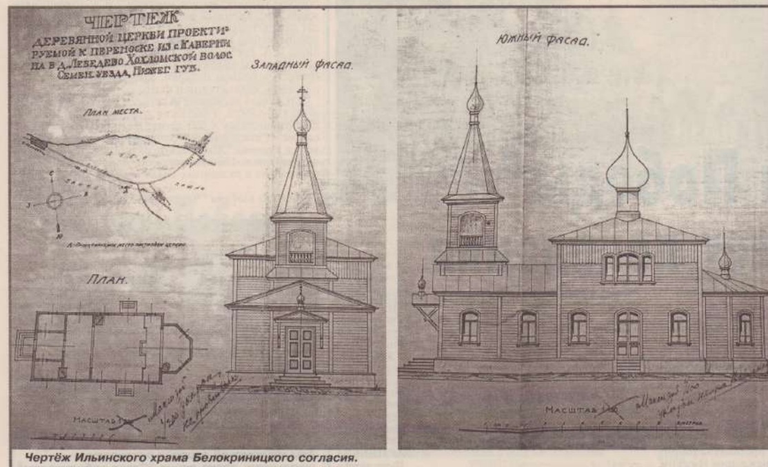
Чертеж Ильинского храма Белокриницкого согласия.
