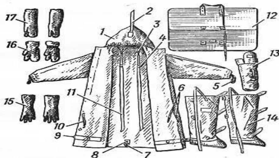
Рис. 6.1. Общевойсковой защитный комплект: 1 — защитный плащ ОП-1М; 2 — затяжник; 3 — петля спинки; 4 и 7 — рамки стальные; 5 — петля для большого пальца руки; 6 и 10 — закрпки; 8 — центральный шпенец; 9 — хлястик; 11 — держатели плаща; 12 — чехол для защитного плаща ОП-1М; 13 — чехол для защитных чулок и перчаток; 14 — защитные чулки; 15 — защитные перчатки БЛ-1М; 16 — утеплительные вкладыши к защитным перчаткам БЗ-1М; 17 — защитные перчатки БЗ-1М
