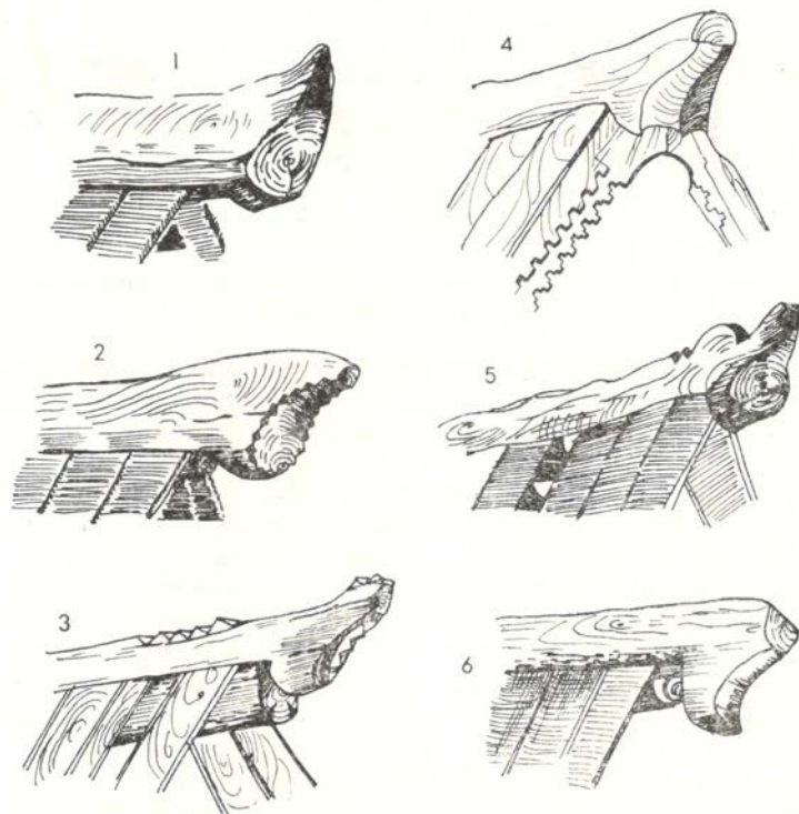
Рис. 2. Охлупни-коньки изб (1, 2, 4—6) и охлупень-конек старого амбара (3) (по Ащепкову) 18 . Рис. М. И. Авдеевой. 1, 2, 4, 5 — д. Язвая, 6 — д. Фыркал Восточно-Казахстанской обл., 3 — д. Брюхановское Томской обл.
