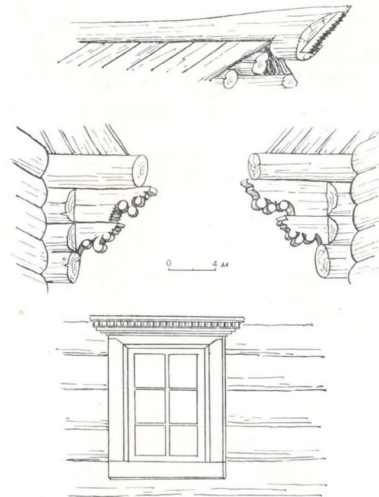
Рис. 6. Охлупень-конек, повалы, окно дома Вдовина в г. Братске (по Маковецкому) 24 . Рис. Т. Ю. Фомичевой.
