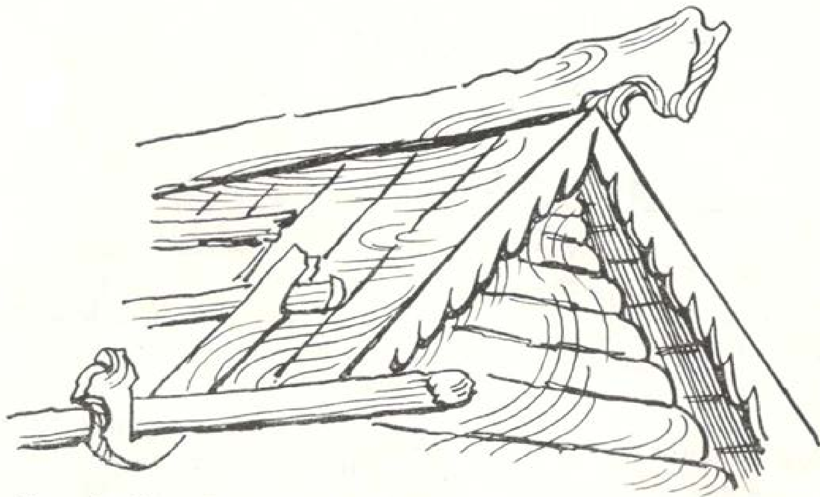
Рис. 8. Крыша на потоках и курицах (по Ащепкову) 27 . Рис. Т. Ю. Фомичевой.
