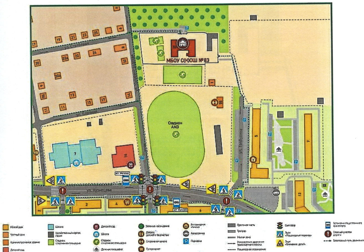
План-схема района расположения МБОУ «С(К)ОШ № 83 г. Челябинска», пути движения транспортных средств и детей
