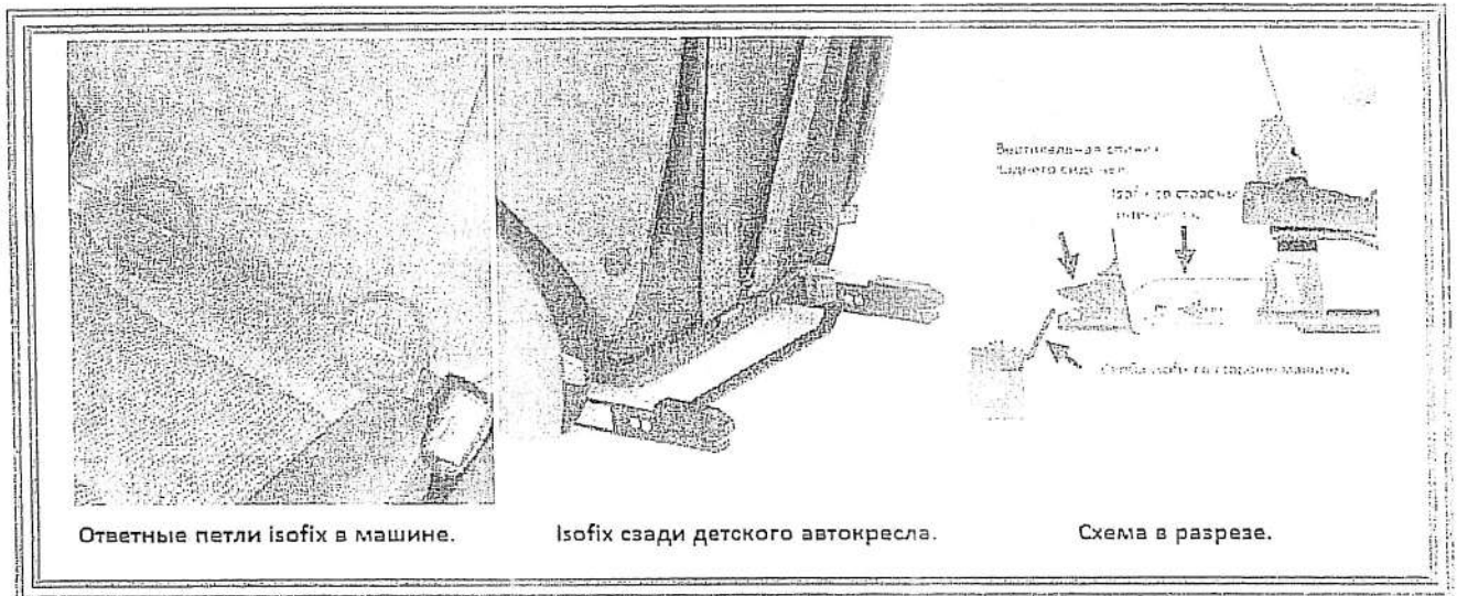
Рисунок 5. Крепления ISOFIX
