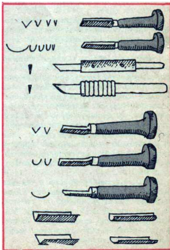
Рис. 15. Резцы
