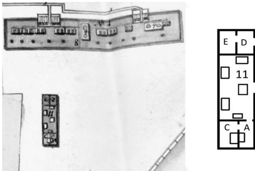
Рис. 4. Фрагмент плана Барнаульского завода начала 1800-х гг. Показана планировка первой плавильной фабрики и кузницы [4, л. 5]. Справа – прорисовка по чертежу. Пояснения обозначениям: А – слесарня, С – инструментальная, D – командная, Е – гиттен-шрейберская.
