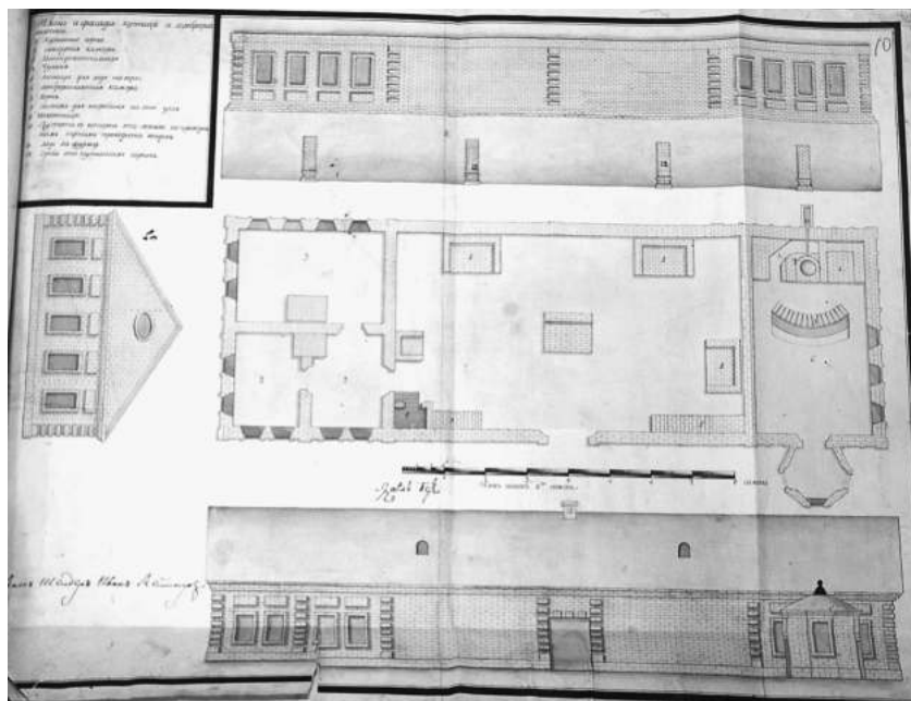
Рис. 2. «План и профиль кузницы Барнаульского завода». Около 1800 г. [6, л. 10].
