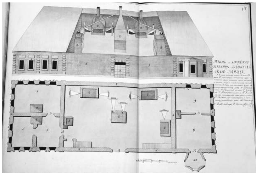
Рис. 3. «План и профиль кузницы Барнаульского завода». Автограф: Берг-мейстер 8-го класса Фролов. 1803–1805 гг. [6, л. 14]
