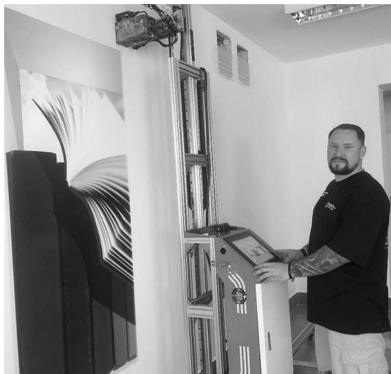
Вертикальный робот-принтер позволяет наносить изображение на любую поверхность.
