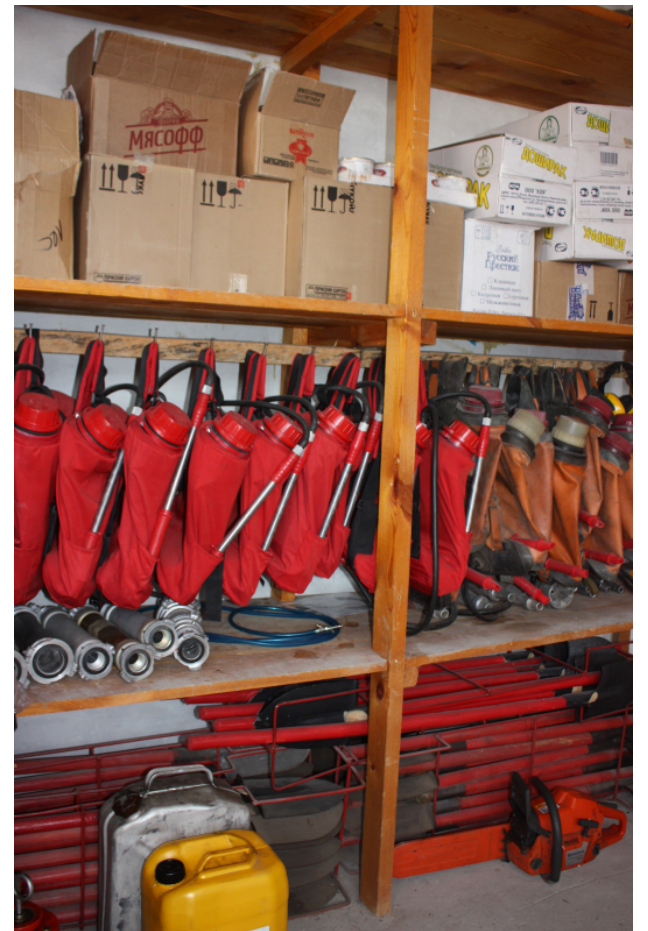
Средства и оборудование для тушения лесных пожаров.
