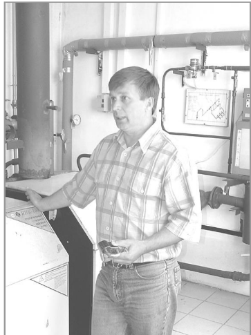
Работники АУ «Альтернатива» готовят котел для установки в Хайрюзовском детском саду.
