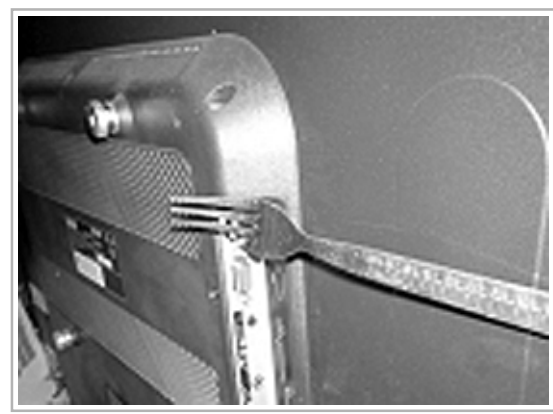
Такую антенну из столовой вилки обнаружили связисты у зрителя, который жаловался на пропадание сигнала. После замены приемной антенны проблемы исчезли.
