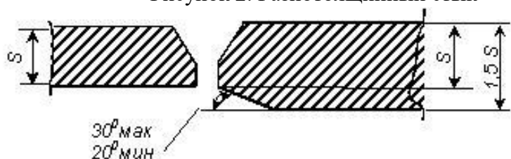
Рисунок 2. Разнотолщинный стык
