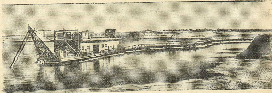
Сталинградгидрострой. Коллектив строителей сооружает котлован под здание Сталинградской ГЭС. Мощные земснаряды вынимают грунт со дна котлована и одновременно намывают ограждающие перемычки.
