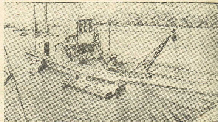
Землесосный снаряд «300-40» № 23 в забое на рытье канала и намыве верхней перемычки котлована Каховской ГЭС.
