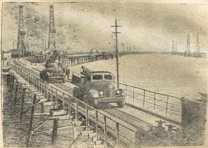
Азербайджанская ССР. С каждым годом расширяется самый молодой в республике морской нефтяной промысел «Нефтяные камни» объединения «Азнефть». На десятки километров протянулась в море стальная эстакада со множеством ответвлений. На них стоят нефтяные вышки.
