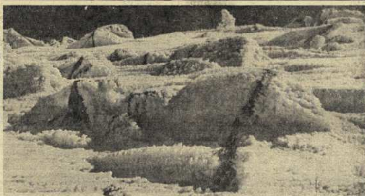
Снежные заструги; любитель походов шахтоострель Н. Федотовский.
