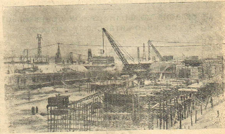
На снимке: общий вид строительства судоходного шлюза Камской ГЭС.
