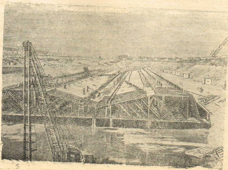
На снимке: общий вид бетонированных блоков днища камер нижнего судоходного шлюза.
