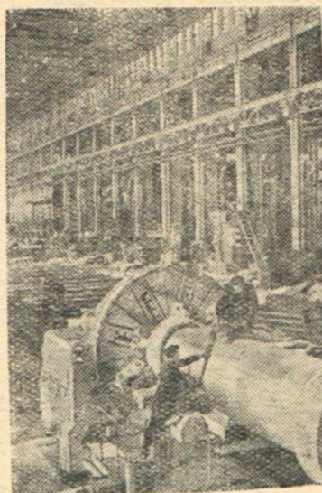
пусе Новосибирского турбогенераторного завода. На переднем плане обработка восьмиметрового вала ротора гидрогенератора для Иркутской ГЭС.
