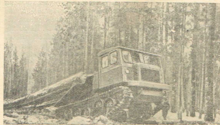
Белорусская ССР. В Бегомльском лесопромхозе широко используется трелевочный трактор «ТТ-54», созданный Минским тракторным заводом. Он снабжен дизельным двигателем мощностью в 54 лошадиных силы. Его грузоподъемность — до 15 кубометров леса. Это почти в два с половиной раза больше, чем грузоподъемность газогенераторного трактора «КТ-12». Трактор оборудован гидравлическими механизмами, облегчающими погрузку леса.
