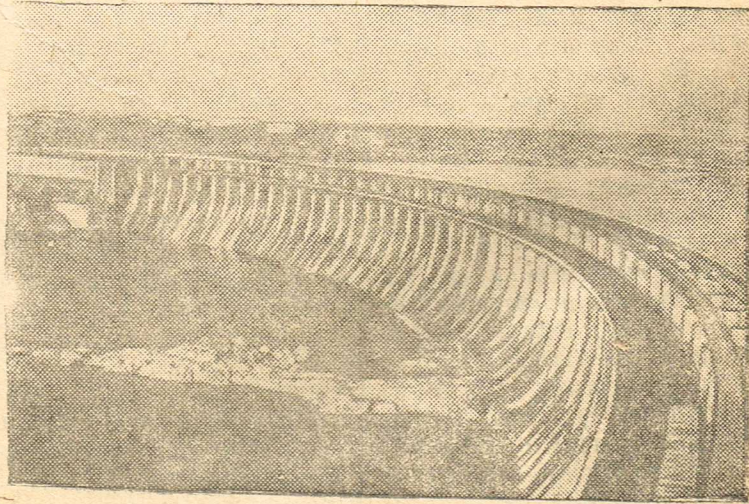
Запружье. Возрожденная плотина Днепровской ГЭС имени Ленина. Фото С. Вильмана. Прессклишэ ТАСС.
