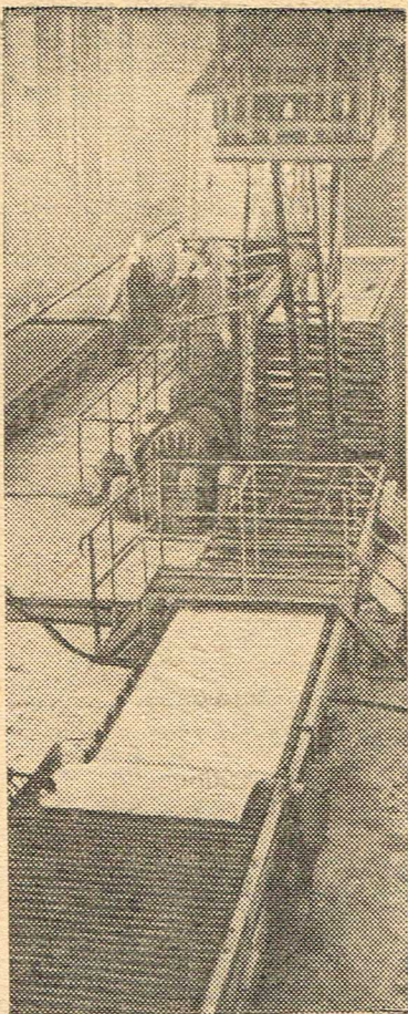
ВОЛЖСК. На Марийском целлюлозно-бумажном комбинате освоено производство древесно-волоконистых плит. Сырьем для их изготовления служит щепа — отходы соседних деревообрабатывающих предприятий.
