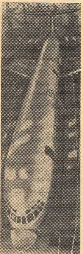
Узбекская ССР. За успешное выполнение плановых заданий и внедрение передовой технологии коллектив Ташкентского авиаремонтного завода гражданской авиации награжден орденом Трудового Красного Знамени.
