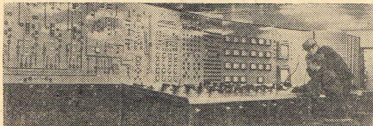
Новолипецкий металлургический завод. С этого пульта, оборудованного новейшими приборами, управляется работа мощной доменной печи.
