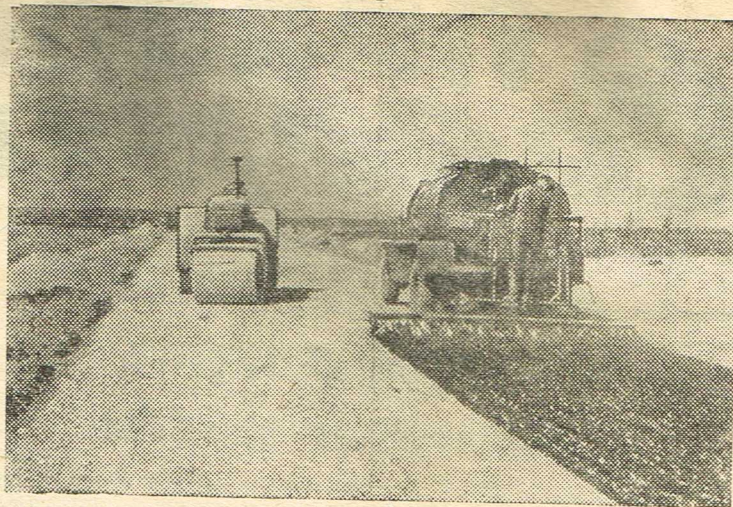
К строительству Куйбышевской гидроэлектростанции от гор. Куйбышева подводится шоссе. На снимке: на трассе строящейся шоссе. Укатка и гидронирование шоссе на стахановском участке производителя работ И. П. Артамошкина.
