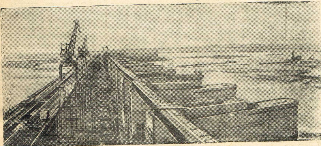
Волгодонстрой. На строительстве Цимлянского гидроузла. С начала заполнения Цимлянского водохранилища уровень Дона около плотины поднимается все выше и выше.
