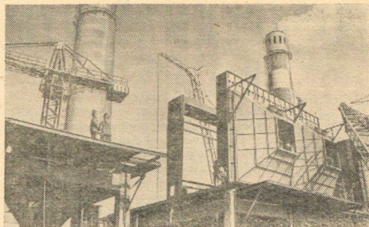
Кантский цементный завод — крупнейшее предприятие строительной индустрии Киргизии. Его первая очередь — две технологических линии — работает на полную мощность. С пуском в эксплуатацию второй очереди предприятие будет давать в год 950 тысяч тонн цемента, 93 миллиона шиферных плиток, большое количество асбоцементных труб.
