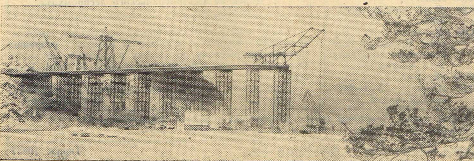
На нижнем снимке: монтаж большой бетоновозной эстакады Усть-Илимской ГЭС. Фото Э. Брюханенко.
