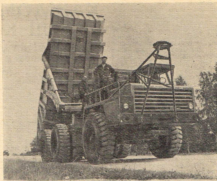
На Белорусском автомобильном заводе изготовлен опытный образец автопоезда-троллейвоза «Белаз-3524». Его грузоподъемность 65 тонн, скорость 50 километров в час. Машина имеет четыре электромотора-колеса, которые получают электроэнергию со стороны через троллейное устройство, а также и от своего генератора, приводимого во вращение дизельным двигателем. Мощность одного электромотора-колеса — 200 киловатт. Автопоезда-троллейвозы найдут широкое применение в угольной и горнорудной промышленности. Сейчас опытный образец проходит заводские испытания. НА СНИМКЕ: автопоезд-троллейвоз «Белаз-3524».
