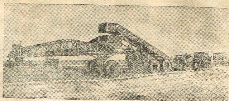
На снимке: Землеройный струг «Д-261», предназначенный для работы на строительстве каналов.
