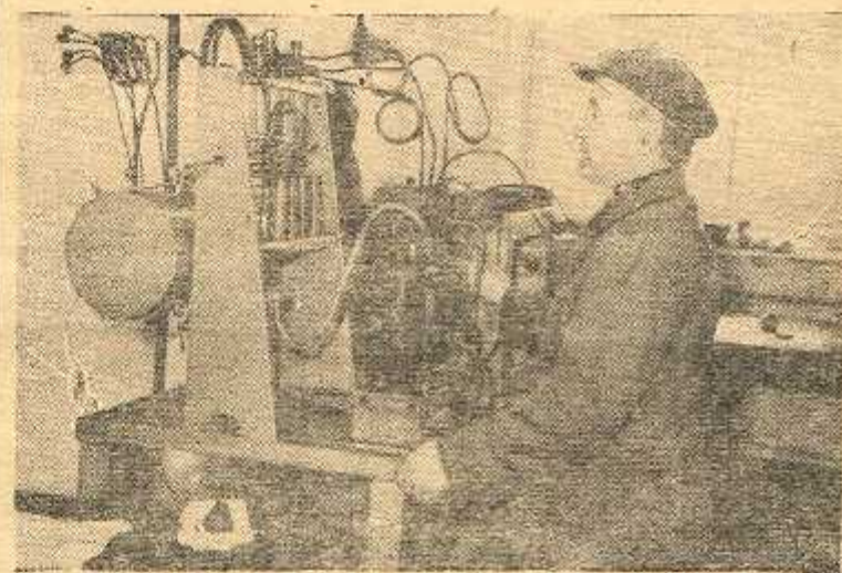
Мастер машинопрокатной базы треста Бокситстрой Л. М. Дворовенко у сделанного им стенда для проверки и регулировки топливной аппаратуры дизелей.
