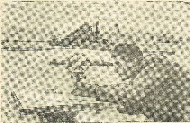
На строительстве Хавовского гидроузла
