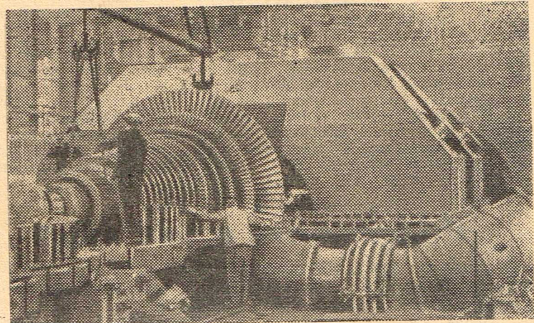
Гигантская паровая турбина мощностью 300 тысяч киловатт, сборка которой показана на снимке, изготавливается Ленинградским Металлическим заводом имени XXII съезда КПСС. Это первая машина для строящейся Конаковской тепловой электростанции, которая будет давать ток системам Мосэнерго и Ленэнерго.
